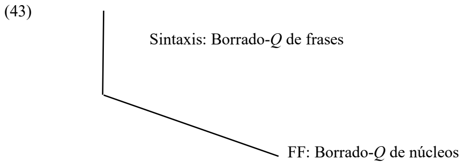
Figura 9. Elipsis derivacional
