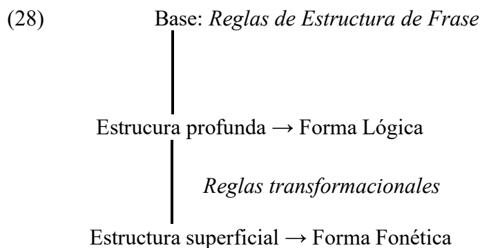
Figura 1. Modelo estándar
