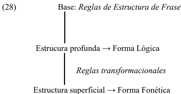
Figura 1. Modelo estándar
