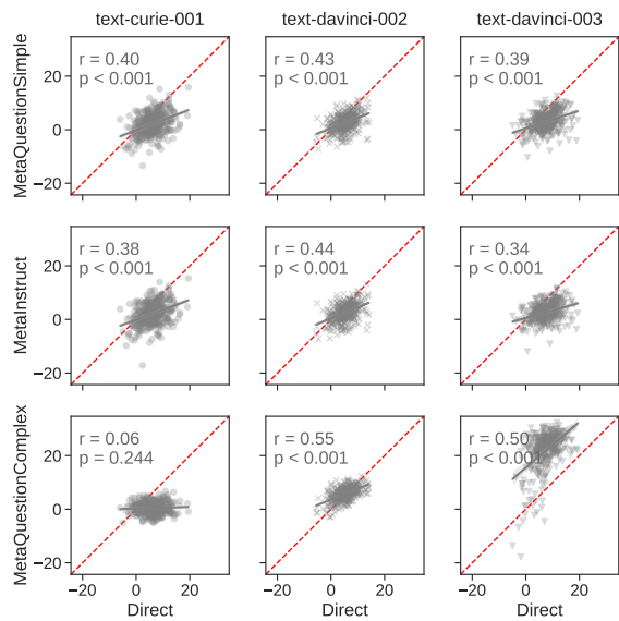
(b) GPT-3*
